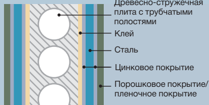
Серийное заполнение ДСП с цилиндрическими отверстиями
