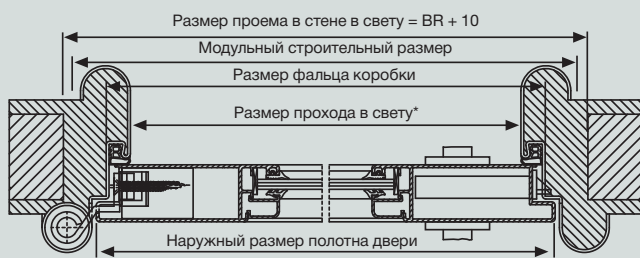
с коробкой «Раундстайл» и петлями «Глобус»
