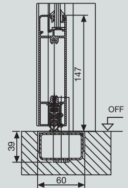
В серийном исполнении без нижнего упора, по желанию с опускаемым уплотнением в основании двери
