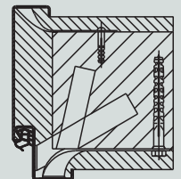
Охватывающая коробка Монтаж в кирпичной/каменной стене Дюбельные анкеры для кирпичной/каменной стены
