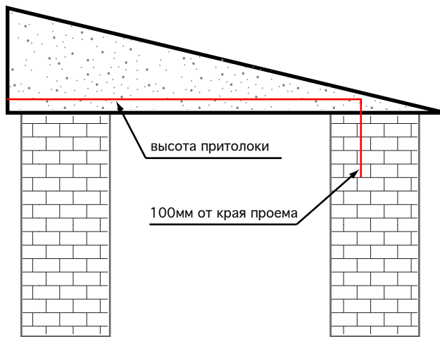
Рис.10 Притолока скошена по ширине проема
