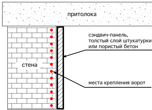
Рис.9 Места крепления ворот к стенам. Вид на правый заплечик изнутри проема
